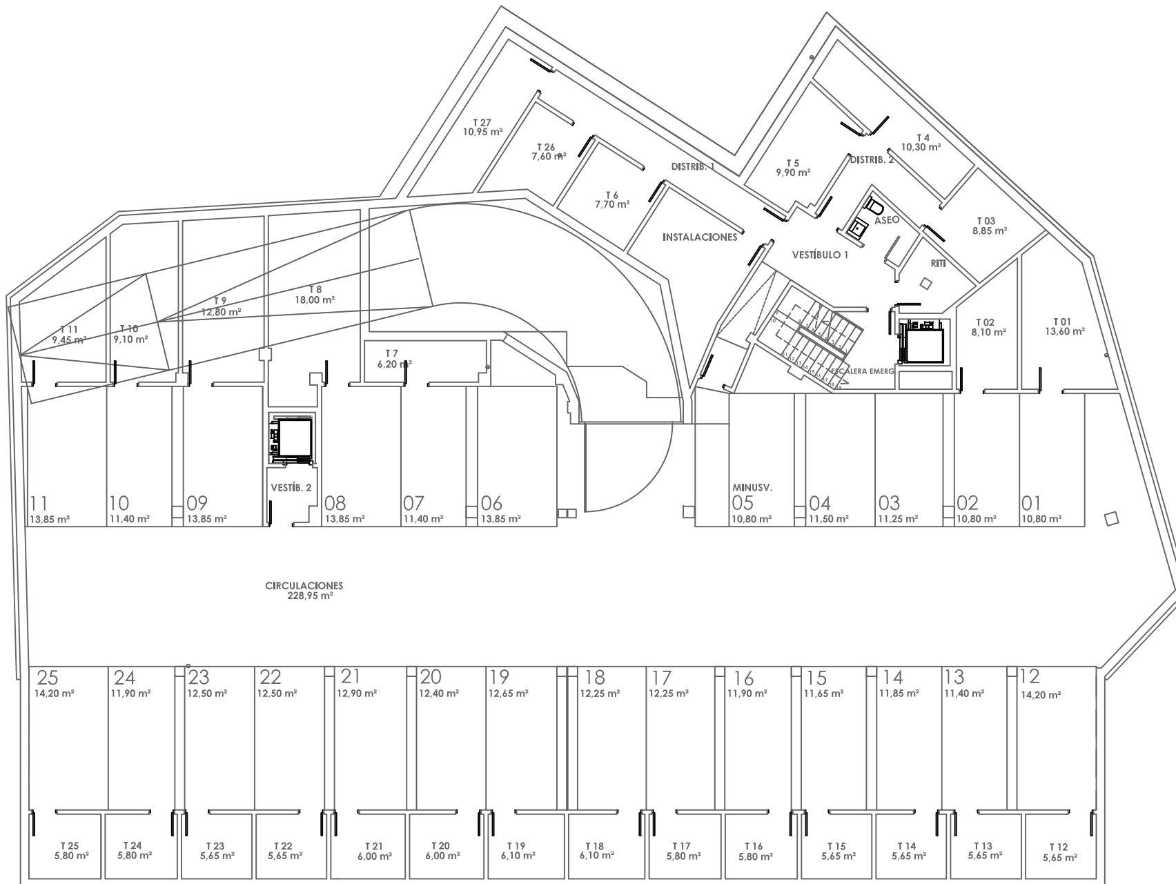
PLANTA SÓTANO
